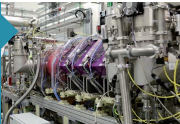
GANIL SPIRAL 2 ACCÉLÉRATEUR DE PARTICULES D'IONS LOURDS
