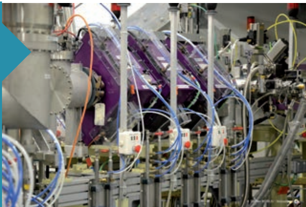
GANIL SPIRAL 2 ACCÉLÉRATEUR DE PARTICULES D'IONS LOURDS
